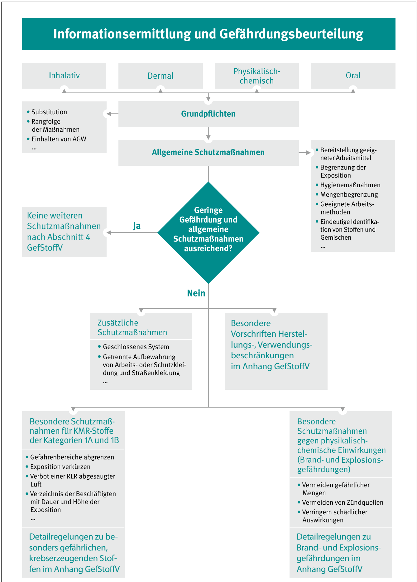
Abbildung 2: Ablaufschema zur Informationsermittlung und Schutzmaßnahmen
