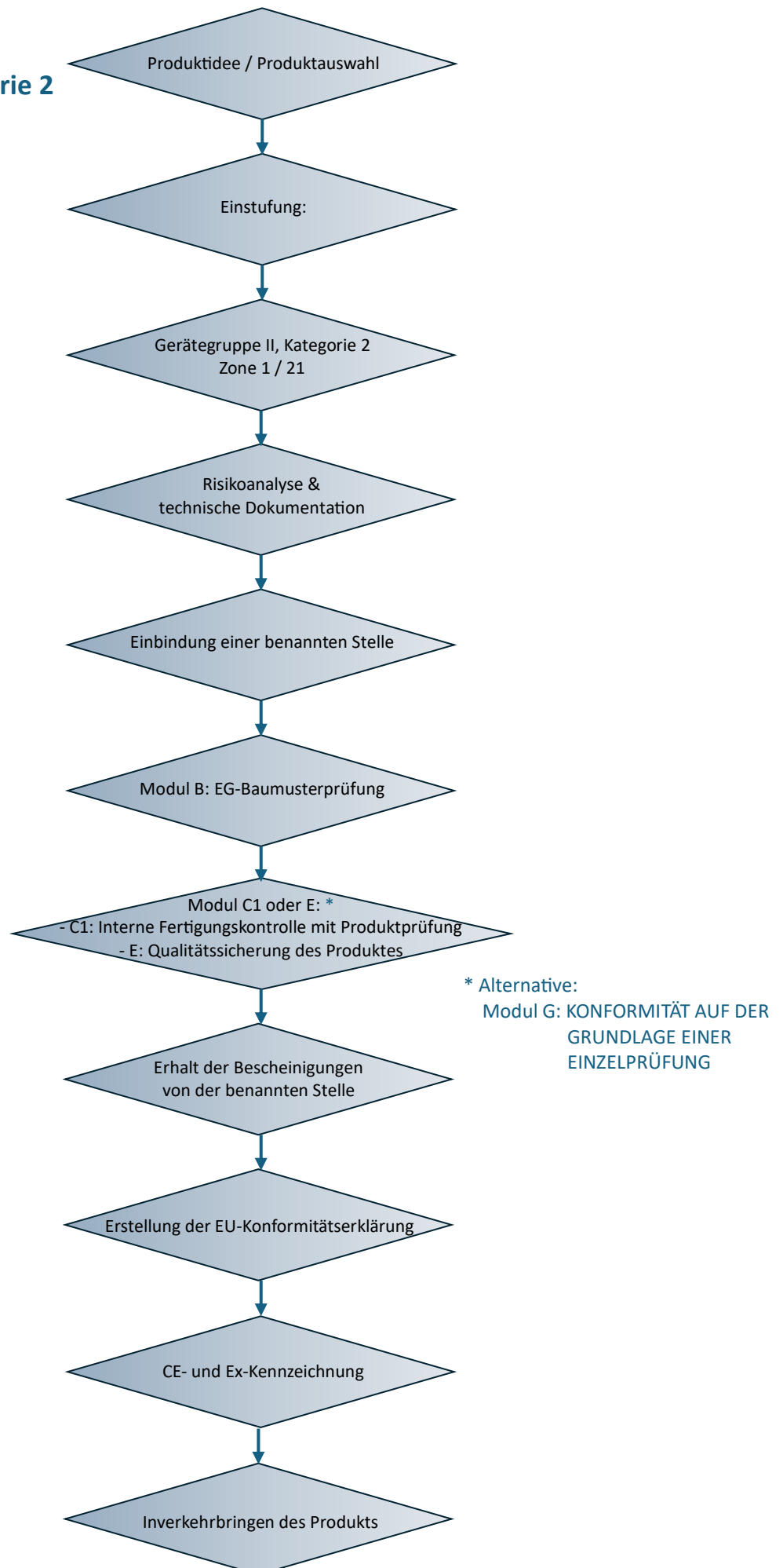
Ablaufdiagramm 2
